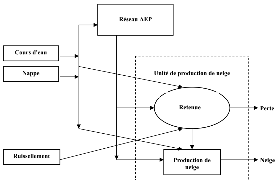
Schéma "entrées – sorties d'eau" des unités de production de neige
